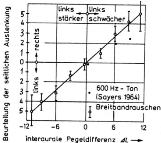
Seitliche Auslenkung des Hörereignisses als Funktion der interauralen Pegeldifferenz. Breitbandrauschen und 600-Hz-Ton, 4 Versuchspersonen, 30 bis 50 Phon.
