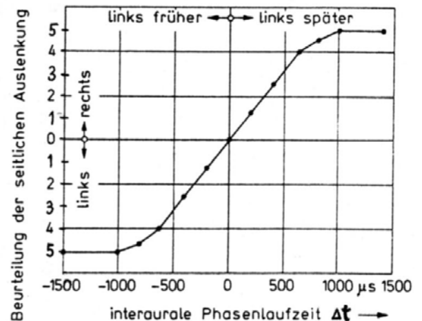
Seitliche Auslenkung des Hörereignisses als Funktion einer verzerrungsfreien interauralen Signalverschiebung. Gültig für Impulse und impulshaltige Signale. 5 Versuchspersonen, Lautstärken von 30 bis 80 Phon unter Verwendung von Meßwerten von TOOLE und SAYERS, 1965
